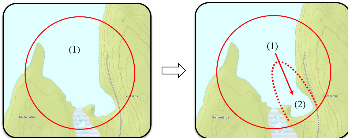
Govus 4. Mohki Seahkka/mohkki (1) namma lea metonymalaččat sirdásan maddái várppi namman Seahkkamohkki (2) (Kártavuodđu: SSR).
