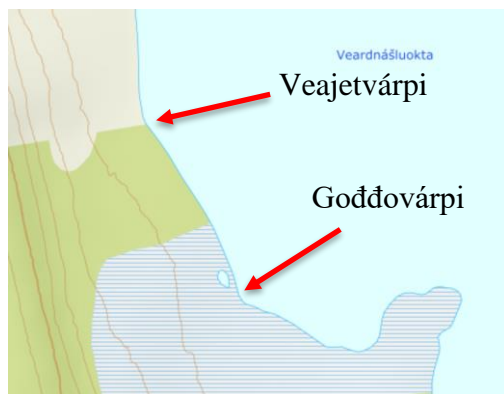
Kárta 6. Godđovárpi ja Veajetvárpi (Kártavuoddu: SSR).
